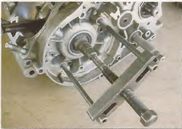
Separador de carcasas
